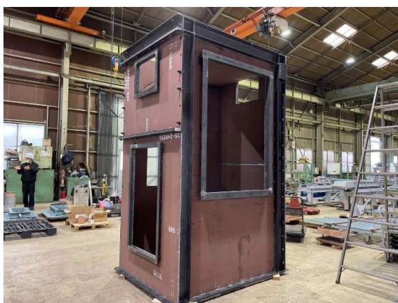
HARDOX500 エレベーターケーシング
