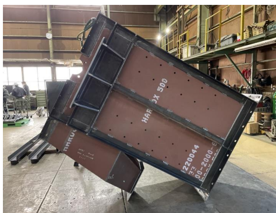
HARDOX500 給鉱ケーシング
