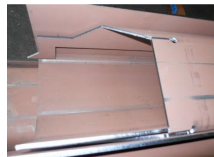
耐摩耗鋼HARDOX450 チャンネル(切欠き)
