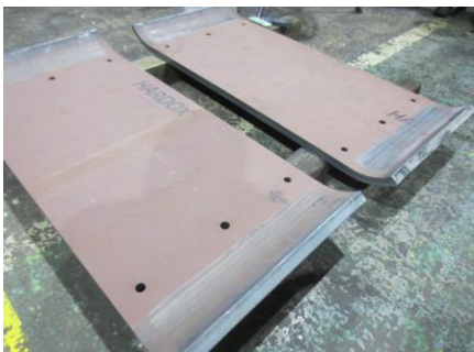
耐摩耗鋼HARDOX500 プレート(25t曲げ加工)
