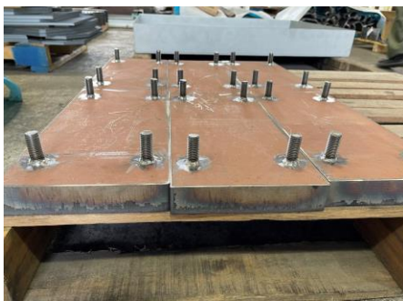
耐摩耗鋼HARDOX500 スタッドボルトライナー
