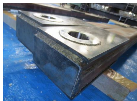
耐摩耗鋼板HARDOX500 パンタグラフ
