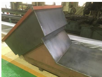
耐摩耗鋼HARDOX450 シュート
