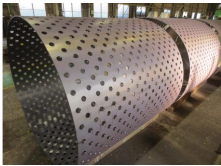
耐摩耗鋼HARDOX500 トロンメル
