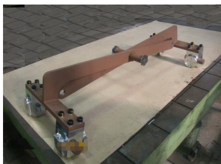
耐摩耗鋼板HARDOX450 シリコン吊り具トンゲ
