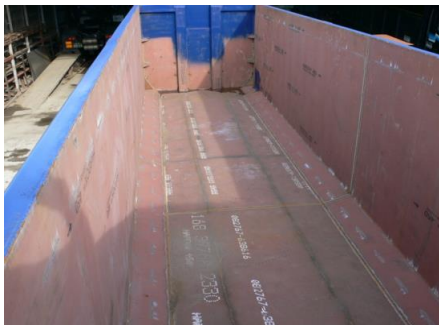
耐摩耗鋼HARDOX450 コンテナ床張り
