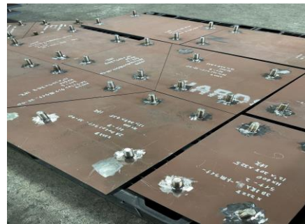
耐摩耗鋼HARDOX600 スタッドボルトライナー
