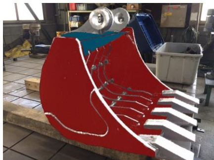
耐摩耗鋼板HARDOX500 スケルトンバケット
