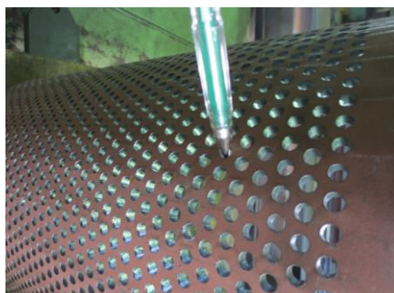
耐摩耗鋼HARDOX450 スクリーン(Φ6穴)
