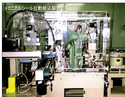
メカニカルシール自動組込装置
