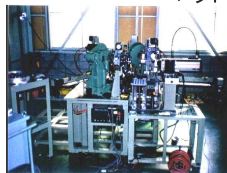
メカニカルシール自動組込装置
