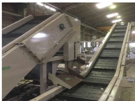
エプロンコンベヤ
