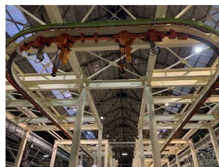
塗装ラインフレーム搬送設備
